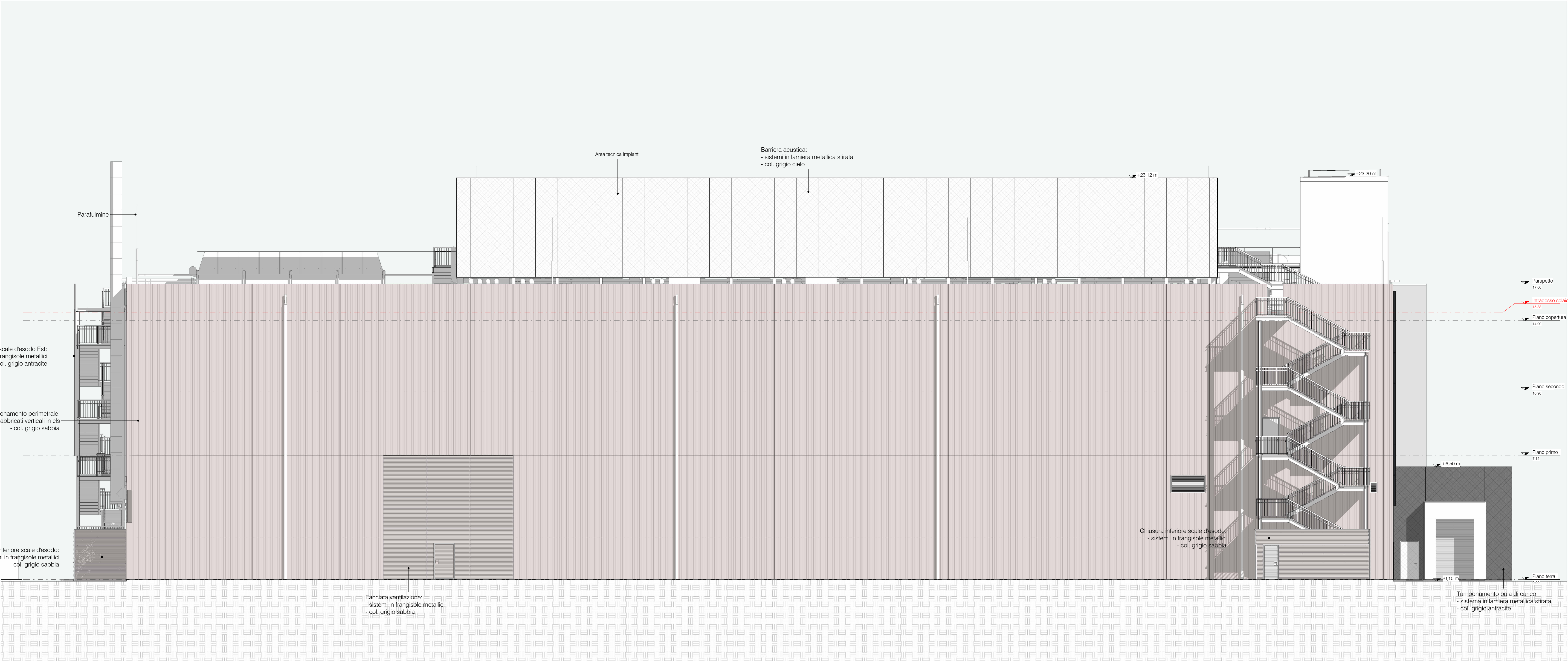
3 Prospetto Nord 1 : 100
