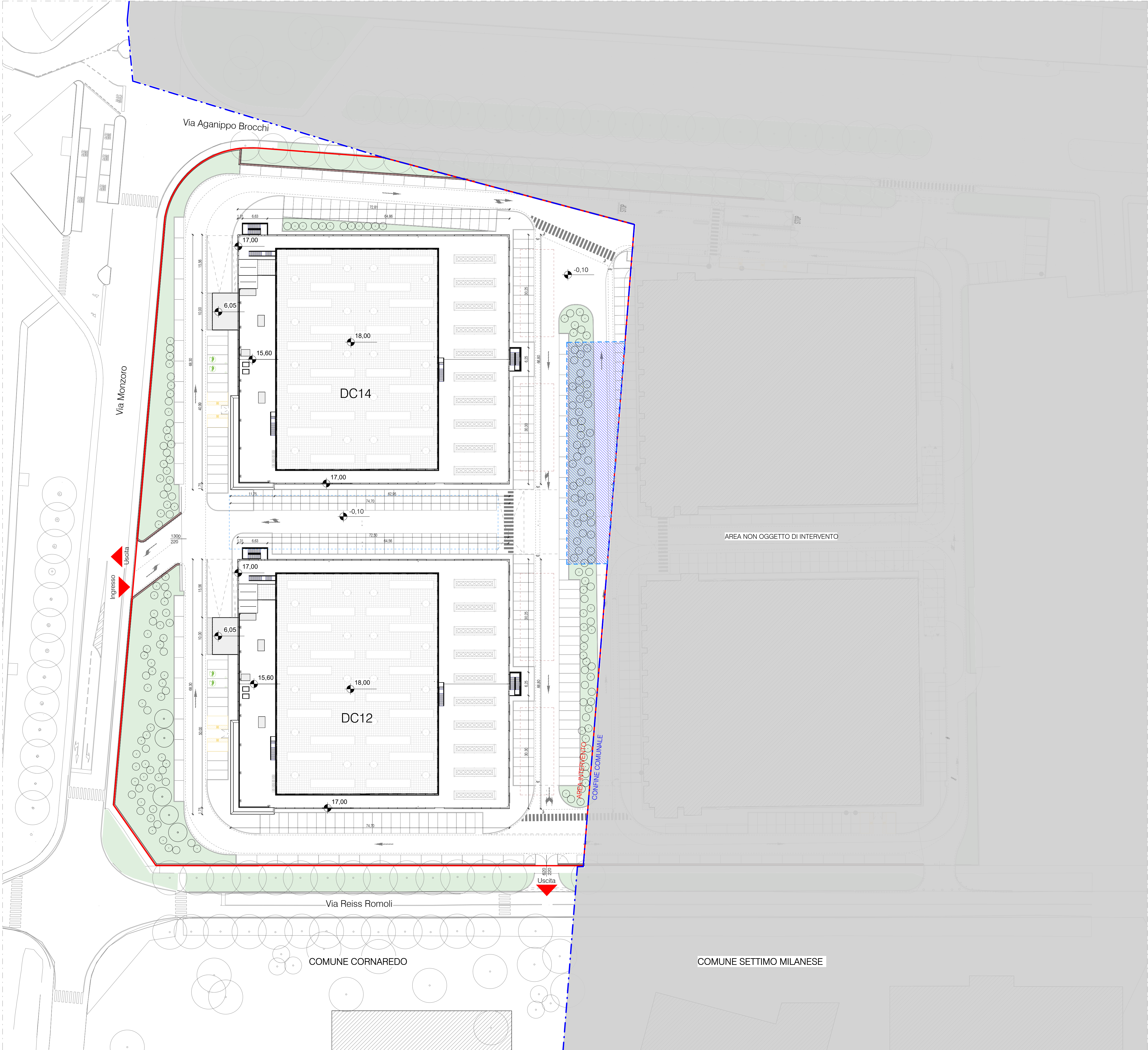
1 Planimetria - Stato Di Progetto 1 : 500
