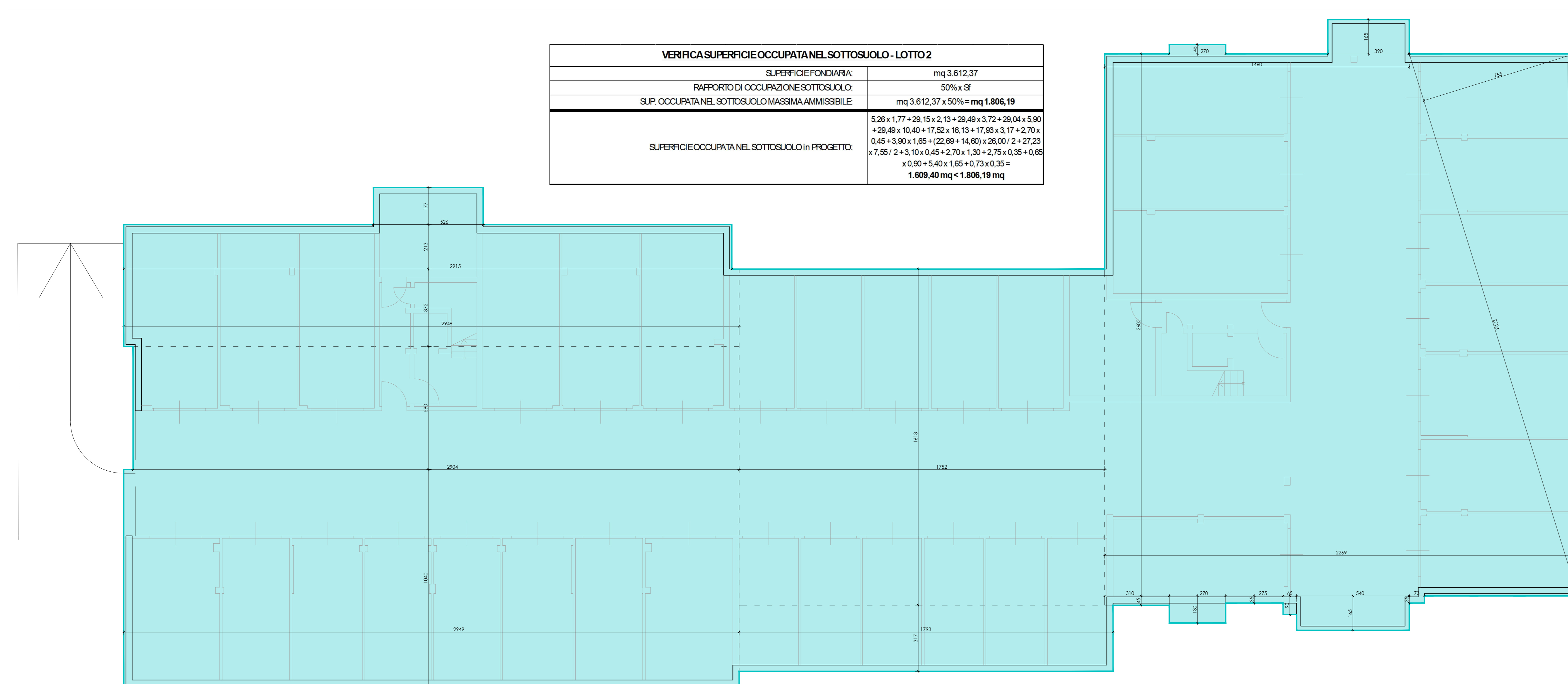
Pianta con indicazione Sup. occupata nel sottosuolo in progetto SCALA 1:100
