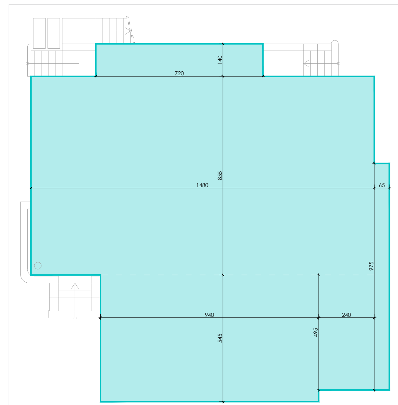
FABB. ESISTENTE - Pianta con indicazione Sup. occupata nel sottosuolo esistente - SCALA 1:100
